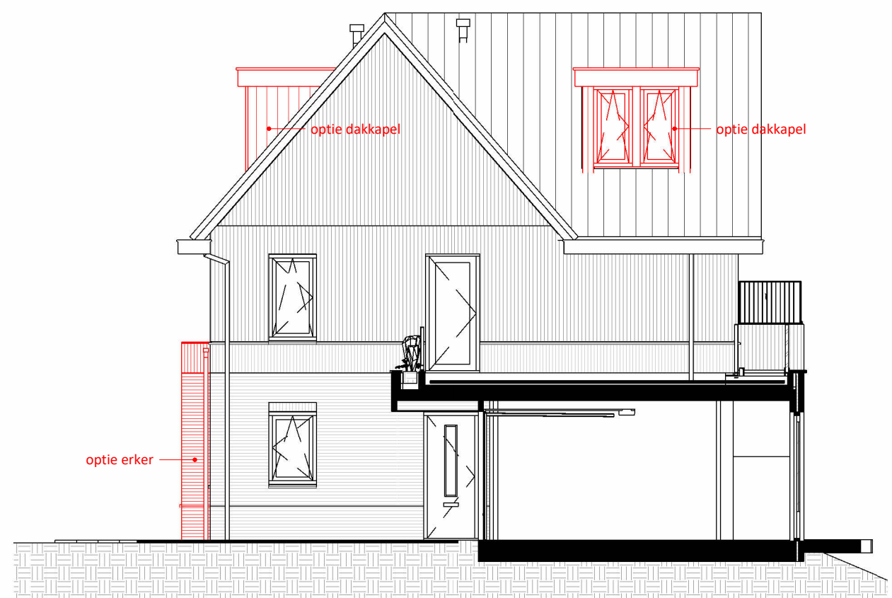
ZIJAAANZICHT BWN. 4 1 : 100
