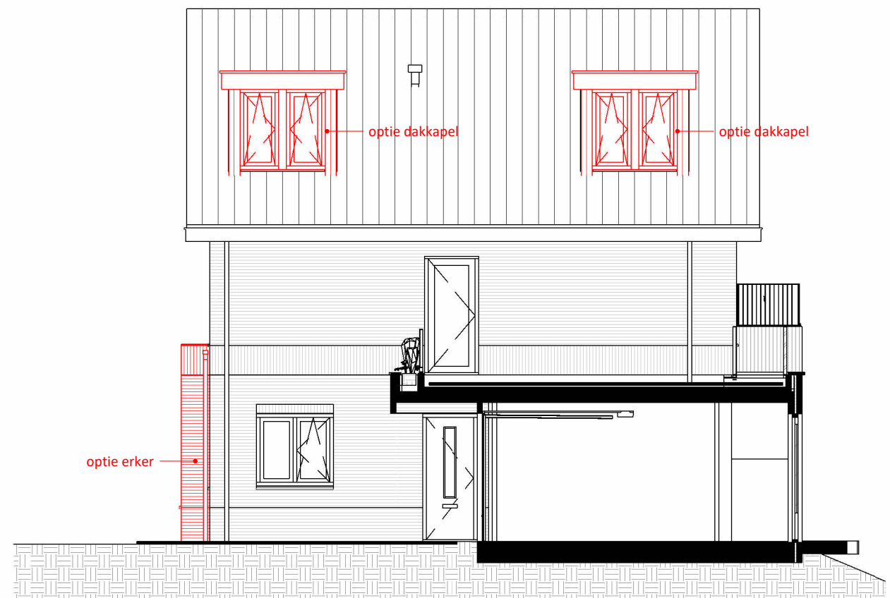
ZIJAAANZICHT BWN. 5 1 : 100
