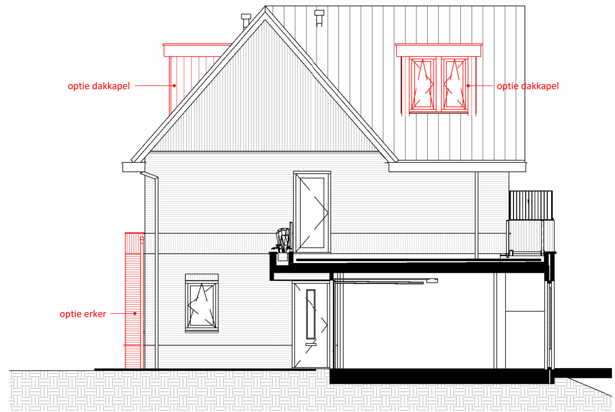
ZIJAAANZICHT BWN. 6 1 : 100
