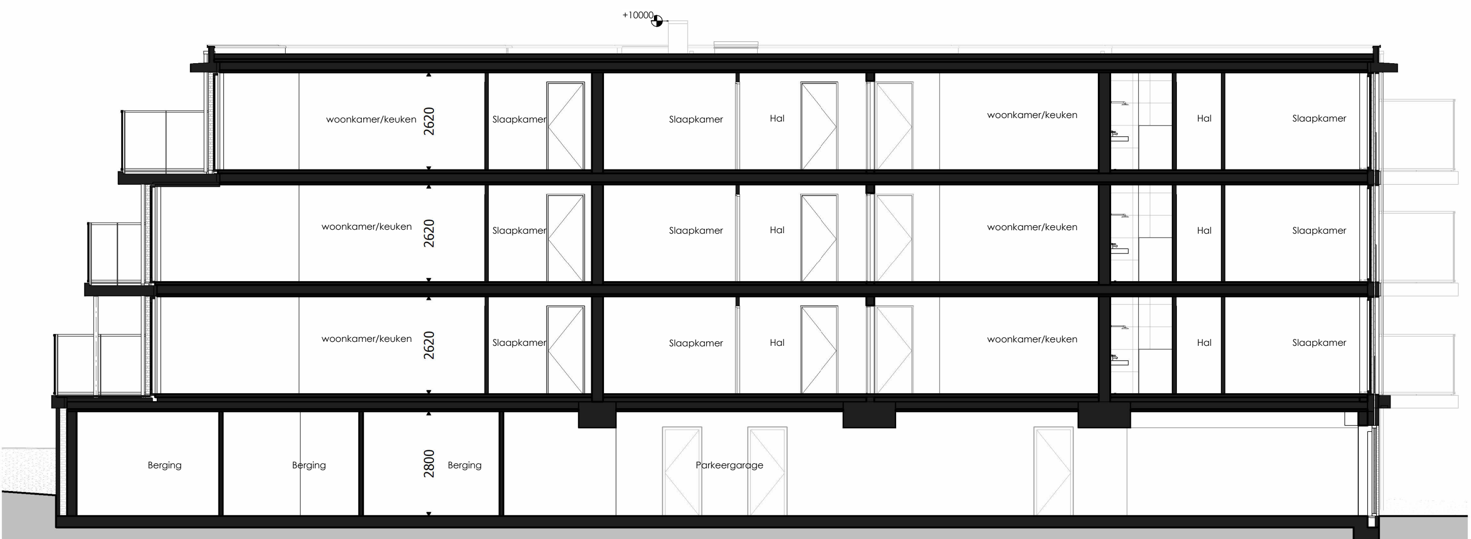
langsdoorsnede
